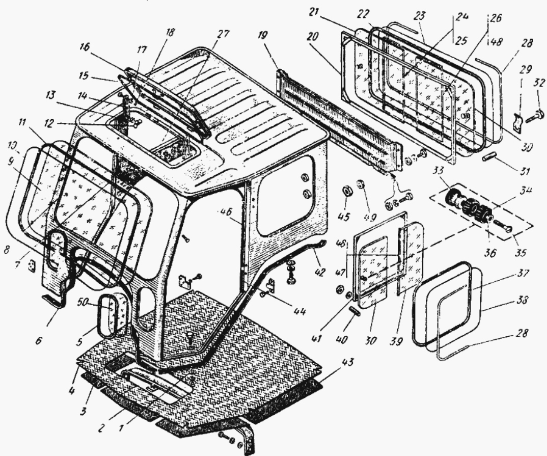
Рис. 65. Рама ветрового окна. Каркас кабины
