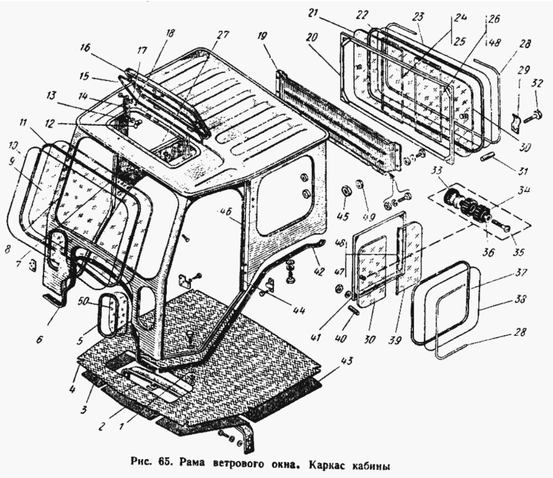
Рис. 65. Рама ветрового окна. Каркас кабины.
